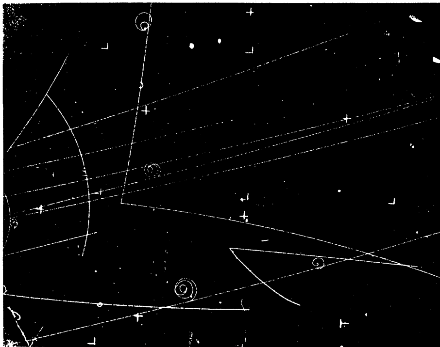
Fig. 1. \pi^- + p \rightarrow K^0 + \Lambda .
