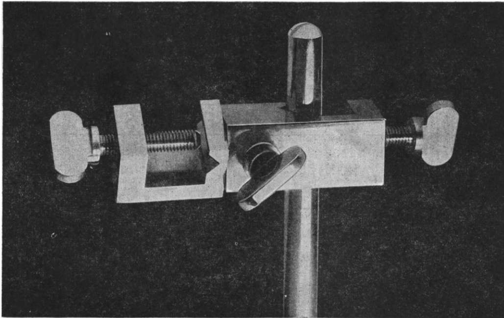
Swivel Clamp—Eleven-tenths Actual Size
