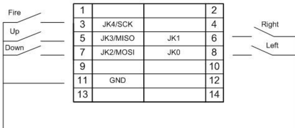
Подключение джойстика
