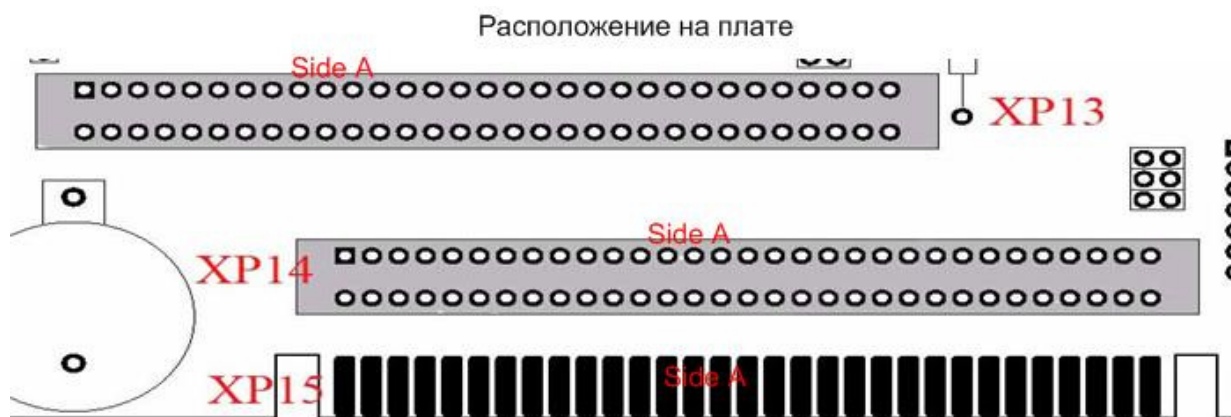
Назначение сигналов
