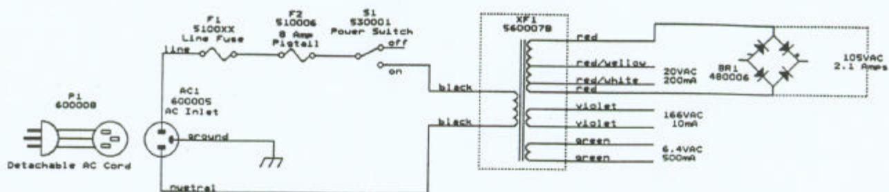
120 VAC WIRING
