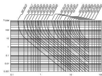
Зависимость времени срабатывания от проходящего тока при t = 23^\circ\text{C} .
