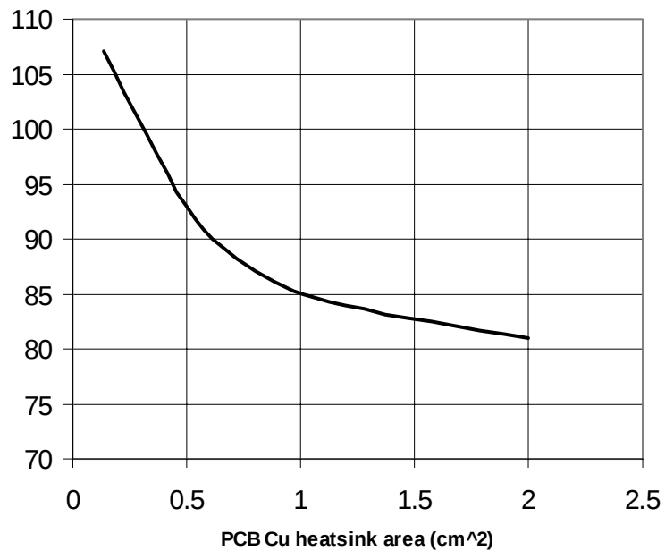
R_{thj-amb} (°C/W) SO-8 at 2 pins connected to TAB
