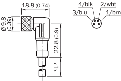
Габаритный чертеж (Размеры, мм)
