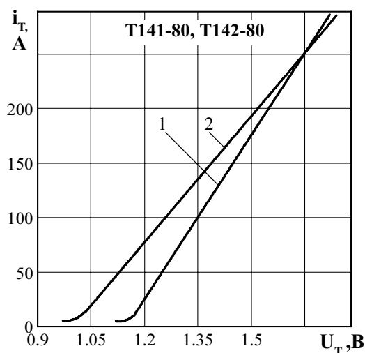
Рисунок 1 - Предельная вольтамперная характеристика в открытом состоянии при температуре перехода 25^\circ\text{C} (1) и максимальной температуре перехода T_{jm} (2) I_T = 3,14I_{T(AV)}
