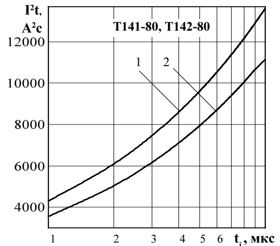
Рисунок 9 - Зависимость защитного показателя I^2t от длительности импульса тока t_i при исходной температуре структуры T_j = 25\text{ °C} (1) и максимальной температуре T_{jm} (2)
