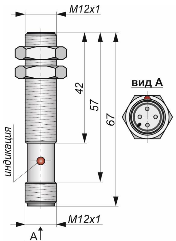
Габаритный чертеж
