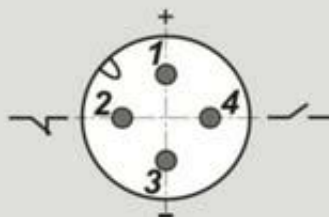
Цоколевка разъема
