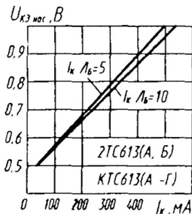
Зависимости напряжения насыщения коллектор—эмиттер от тока коллектора
