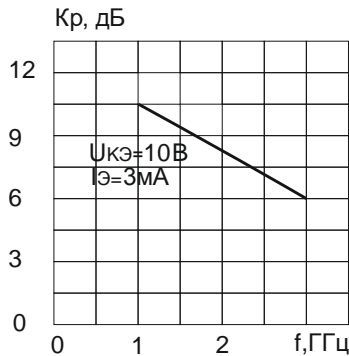
Зависимость коэффициента усиления по мощности от частоты
