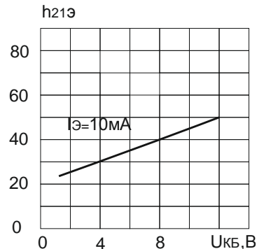
Зависимость статического коэффициента передачи тока в схеме с общим эмиттером от напряжения коллектор-база
