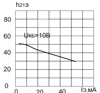
Зависимость статического коэффициента передачи тока в схеме с общим эмиттером от постоянного тока эмиттера
