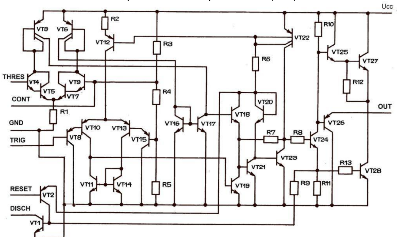
Электрическая схема таймера типа 1006BI1 (Рис.2)
