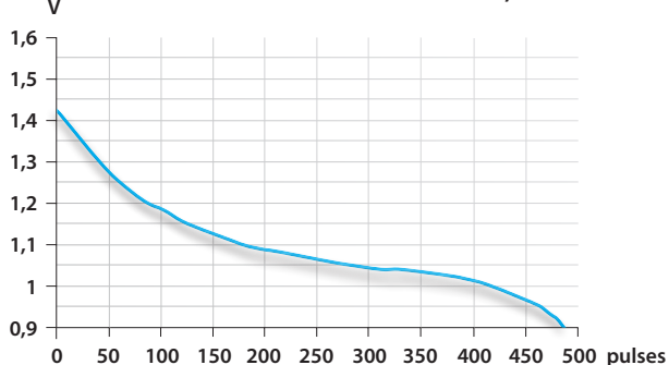
Fotoflash: 10s/m 1h/d 1000 mA end 0,9 V
