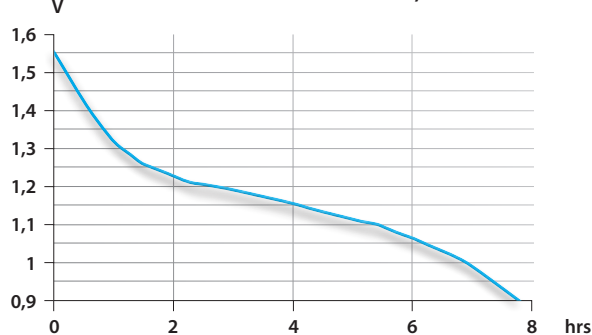
CD/MD: 1h/d 250 mA end 0,9 V
