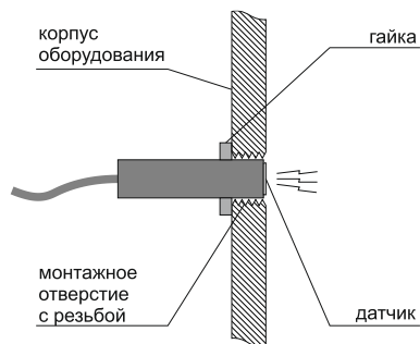
Рисунок 25 - Установка датчика утапливаемого исполнения
