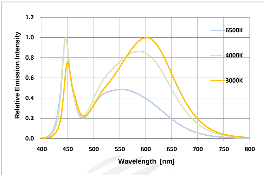
Fig 1-13 Spectrum Distribution光譜分布特性曲线
