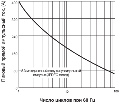
Рис.2 - Максимальный неповторяющийся пиковый ударный прямой ток
