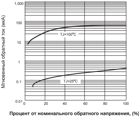
Рис.4 - Типичная обратная характеристика
