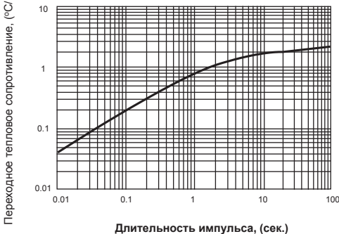
Рис.6 - Типичное переходное тепловое сопротивление
