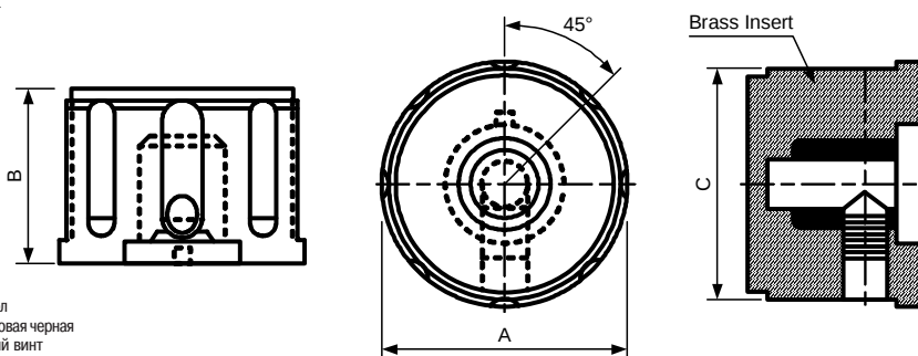
Размеры, мм
