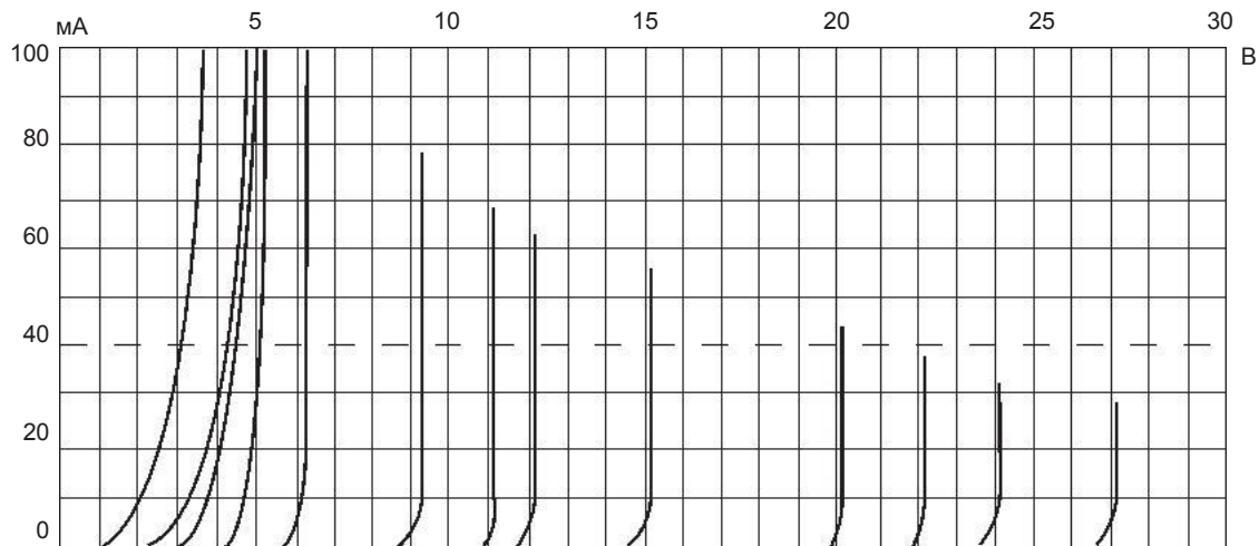
Разгонные характеристики
