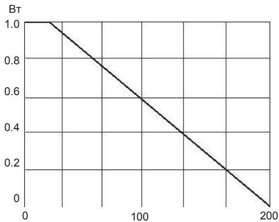
Допустимая мощность рассеяния в зависимости от температуры окружающей среды
