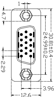
HDB 15M
