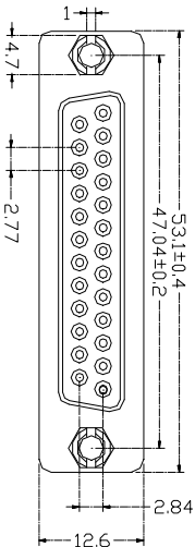
DB25F
