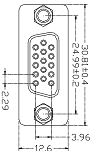
HDB 15F
