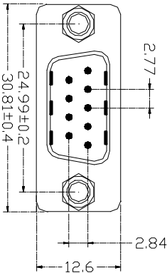
DB9M
