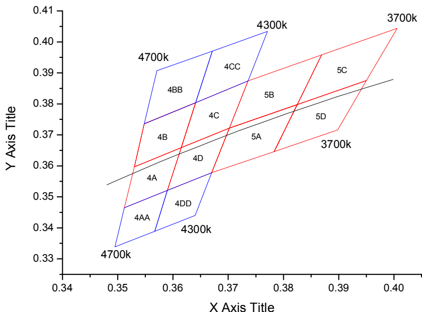
色坐标分档图 Chromaticity Diagram of Ranking
