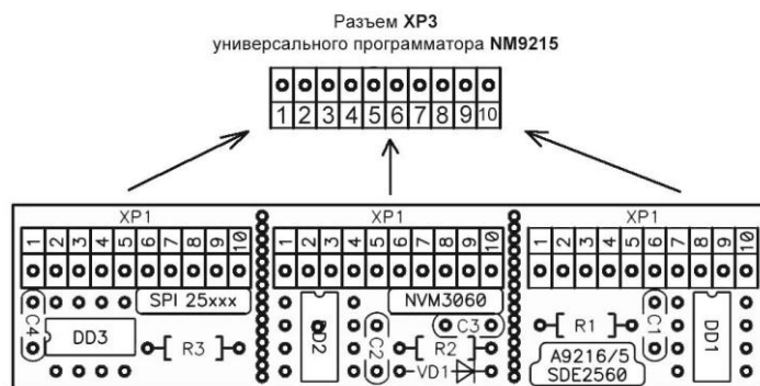
Рис.2 Монтажная схема
