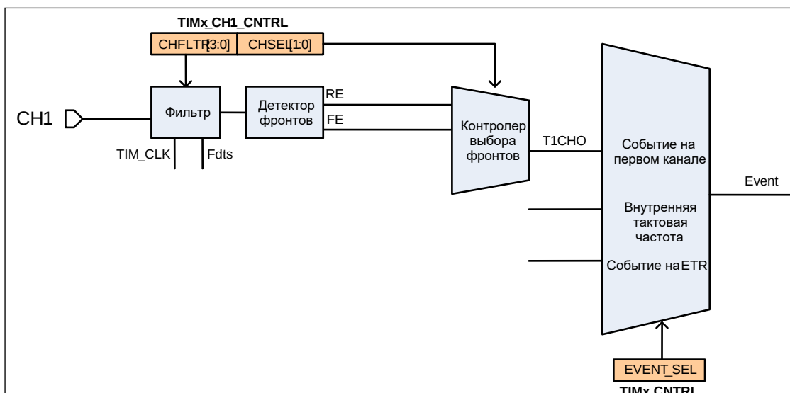
Рисунок 43 – Тактирование с входа первого канала
