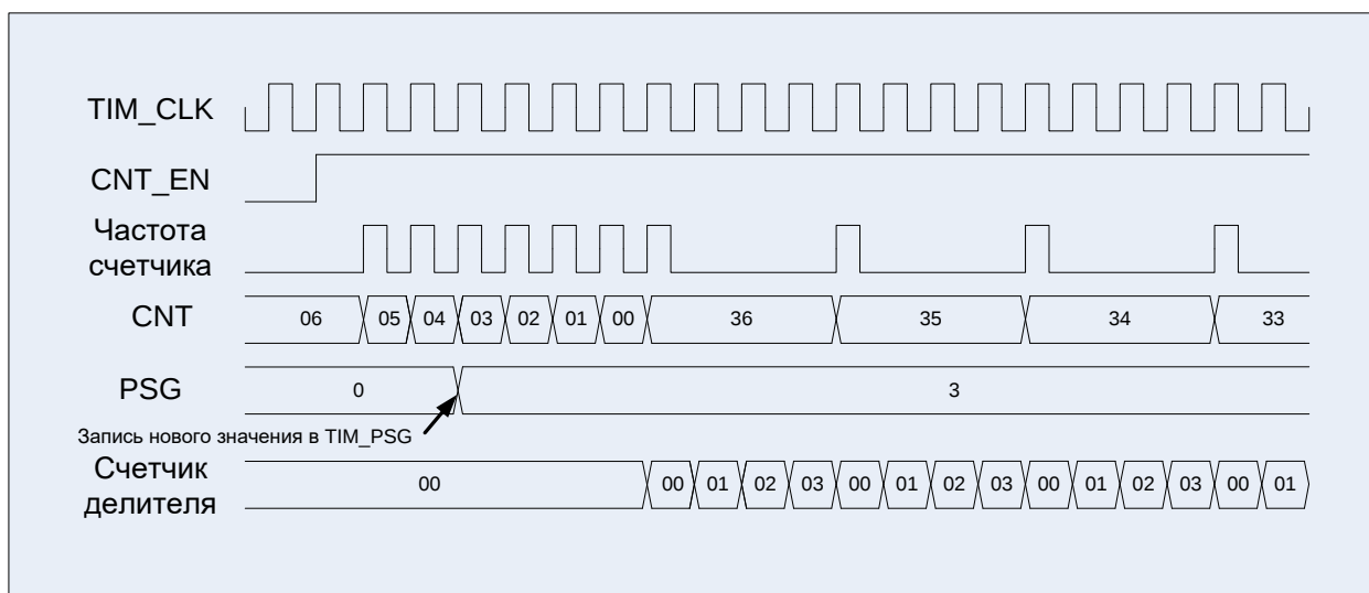
Рисунок 38 – Диаграммы работы счетчика: счет вниз (CNT_MODE = 00, EVENT_SEL = 0000, DIR = 1).
