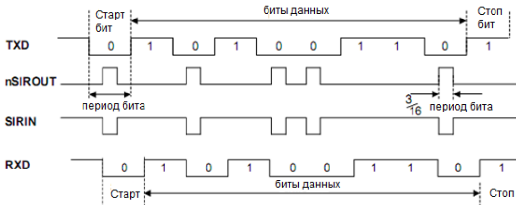
Рисунок 80 – Модуляция данных IrDA
