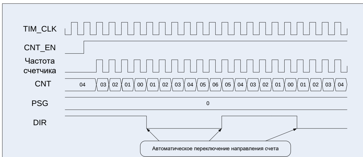
Рисунок 39 – Диаграммы работы счетчика: счет вниз/вверх (CNT_MODE = 01, EVENT_SEL = 0000, DIR = 1).
