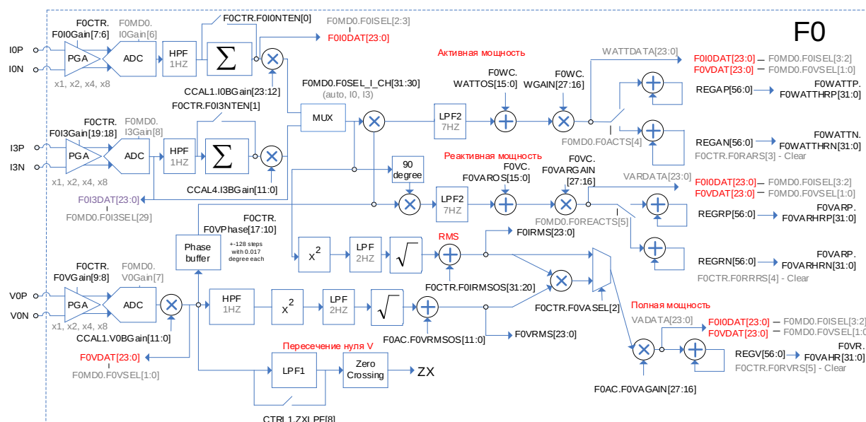
Рисунок 16 – Структурная схема трех каналов АЦП
