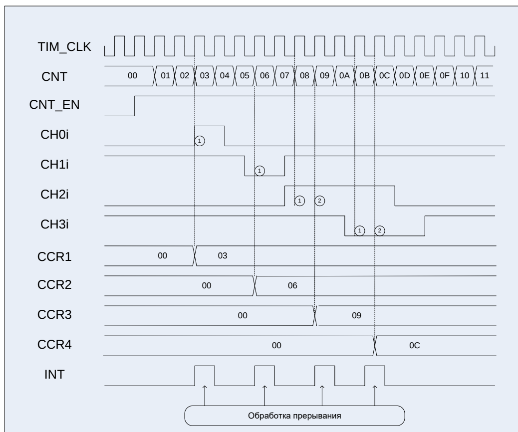
Рисунок 57 – Диаграммы примера работы в режиме захвата
