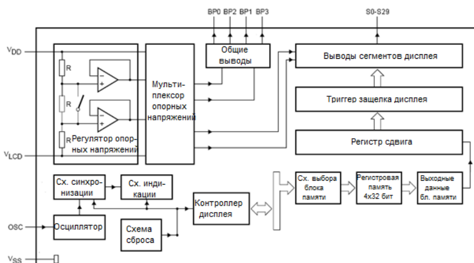
Рисунок 83 – Структурная схема контроллера LCD
