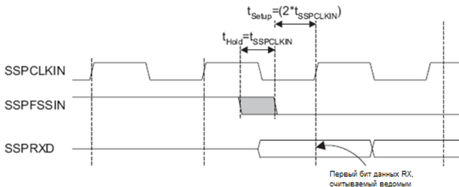
Рисунок 71 – Формат кадра Microwire, требования к времени установки и удержания сигнала SSPFSSIN
