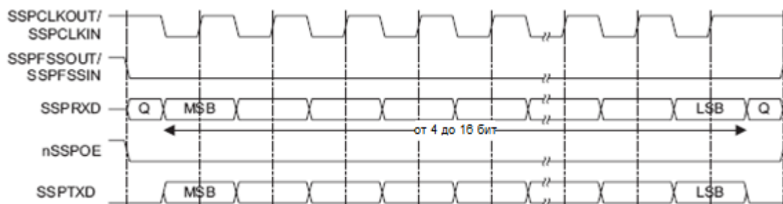
Рисунок 68 – Формат синхронного обмена протокола SPI фирмы Motorola, SPO=1, SPH=1
