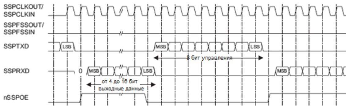
Рисунок 70 – Формат синхронного обмена протокола Microwire фирмы National Semiconductor (непрерывный обмен)
