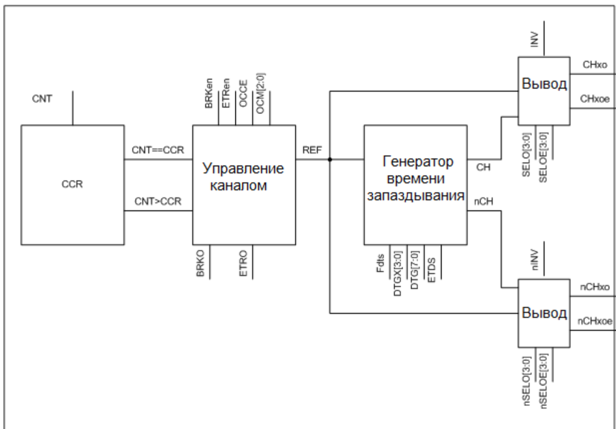
Рисунок 50 – Структурная схема блока сравнения
