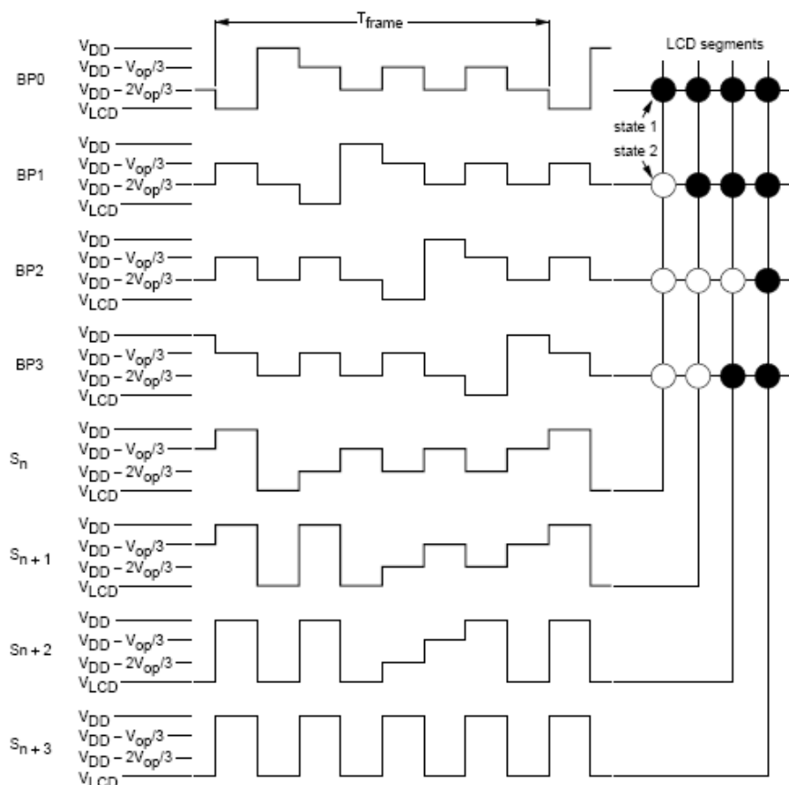
Рисунок 89 – Режим управления с мультиплексом 1:4
