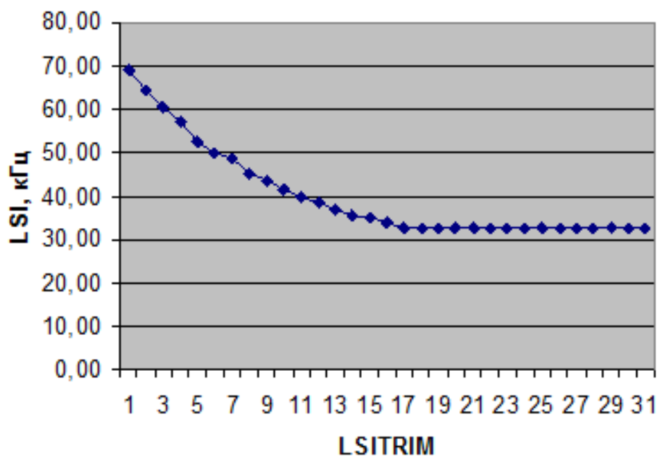
Рисунок 28 – Зависимость частоты LSI от значения LSITRIM
