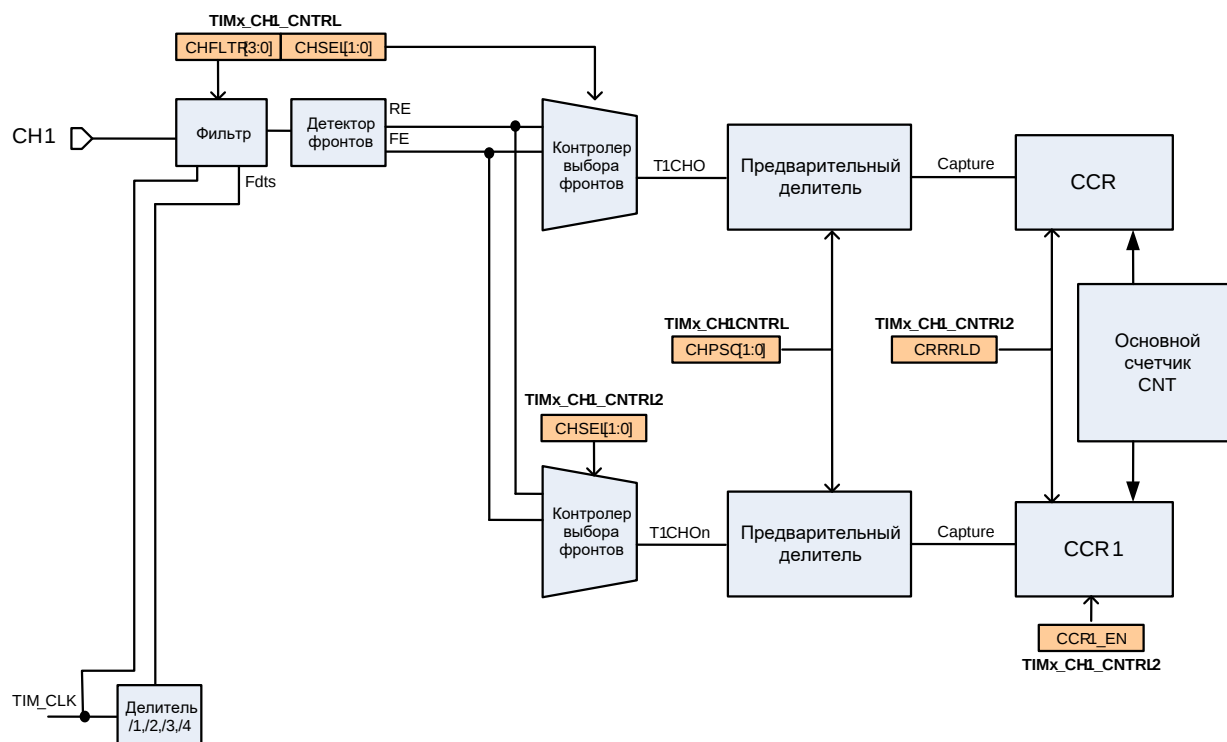
Рисунок 48 – Структурная схема блока захвата на примере канала 1
