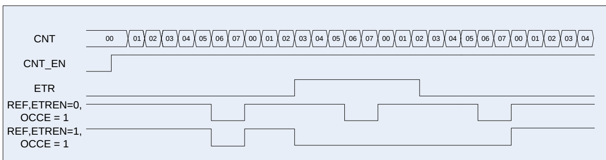
Рисунок 53 – Диаграмма работы схемы в режиме ШИМ, CCR1_EN = 0
