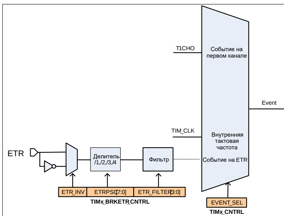
Рисунок 46 – Схема тактирования сигналом со входа ETR
