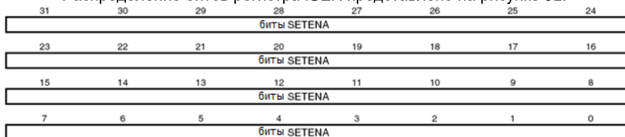
Рисунок 91 – Распределение битов регистра
