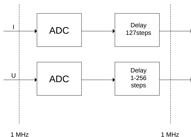
Рисунок 20 – Контролируемый фазовый сдвиг в канале напряжения
