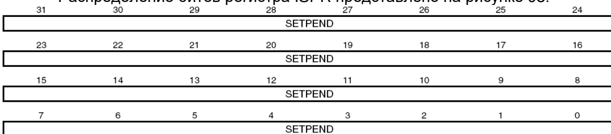
Рисунок 93 – Распределение битов регистра ISPR
