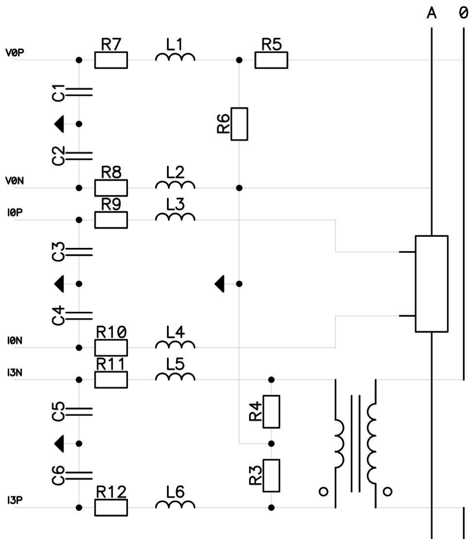
Рисунок 25 – Типовая схема включения для учета электроэнергии по одной фазе с использованием шунта
