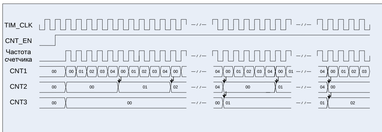
Рисунок 41 – Диаграммы работы двух таймеров в каскаде
