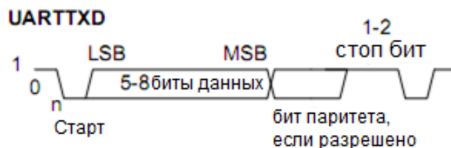
Рисунок 79 – Кадр передачи данных
