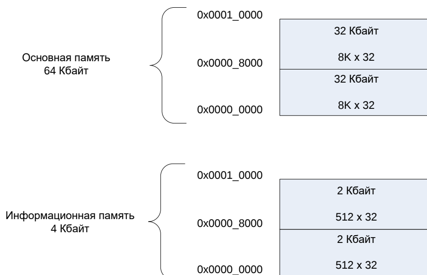
Рисунок 7 – Структура памяти
