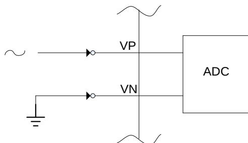
Рисунок 19 – Недифференциальное включение
