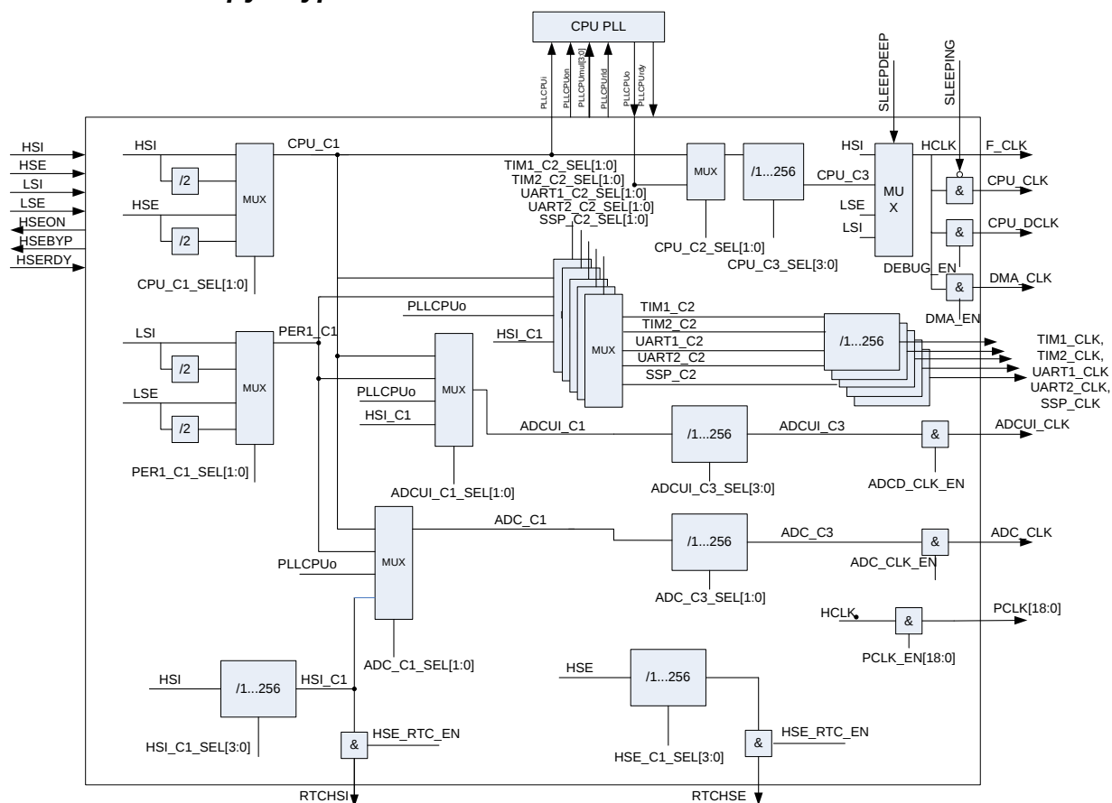
Рисунок 26 – Структурная блок-схема формирование тактовой частоты
