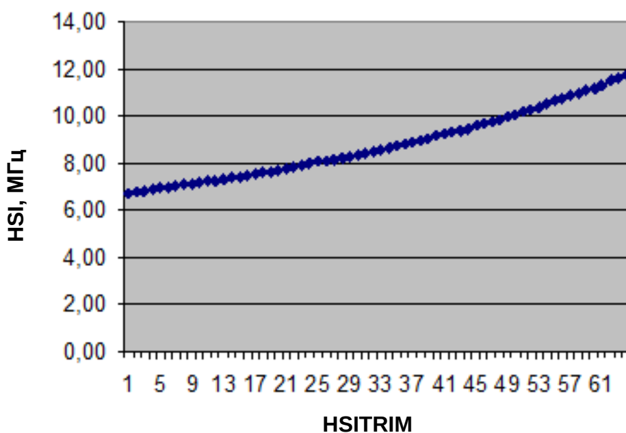
Рисунок 29 – Зависимость частоты HSI от значения HSITRIM
