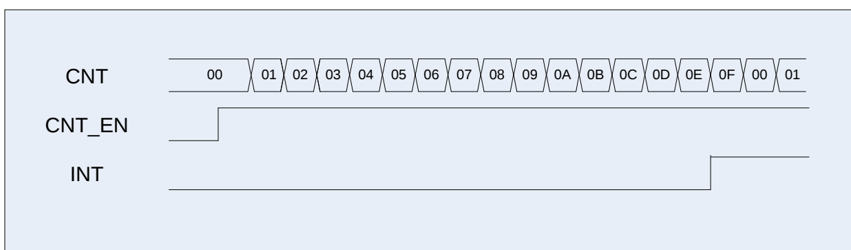
Рисунок 56 – Диаграммы примера работы в режиме обычного счетчика
