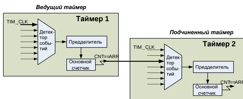
Рисунок 40 – Пример каскадного соединения таймеров
