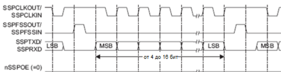
Рисунок 67 – Формат синхронного обмена протокола SPI фирмы Motorola, SPO=1, SPH=0 (непрерывный обмен)
