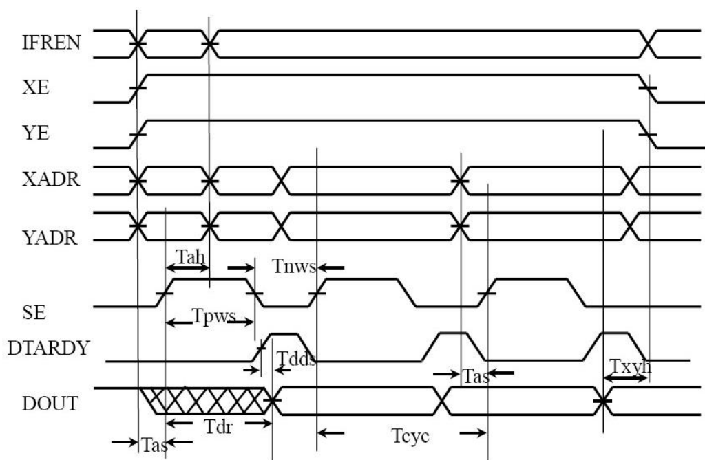
Рисунок 11 – Временная диаграмма чтения памяти
