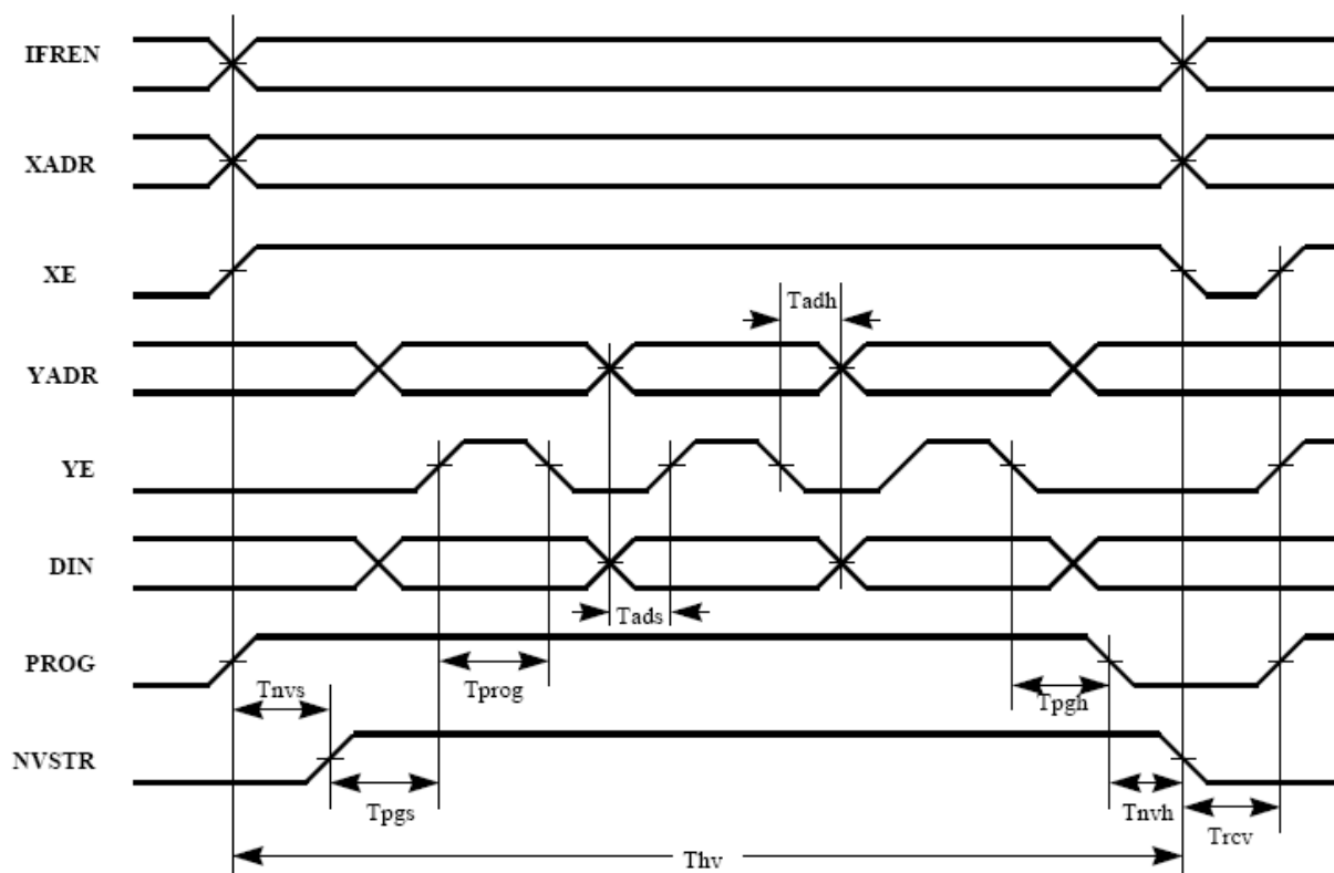
Рисунок 10 – Временная диаграмма записи памяти
