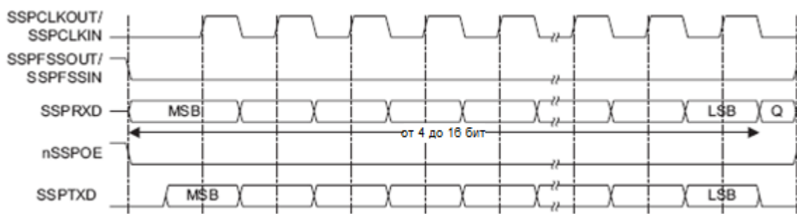
Рисунок 63 – Формат синхронного обмена протокола SPI фирмы Motorola, SPO=0, SPH=0 (одиночный обмен)
