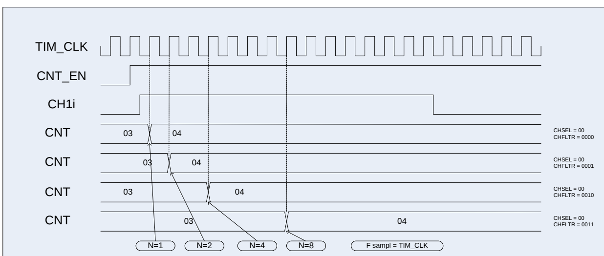
Рисунок 45 – Диаграмма внешнего тактирования с разными вариантами фильтра
