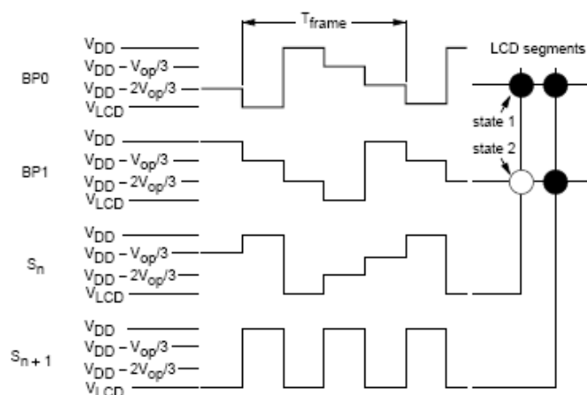
Рисунок 87 – Режим управления с мультиплексом 1:2 и 1/3 bias
