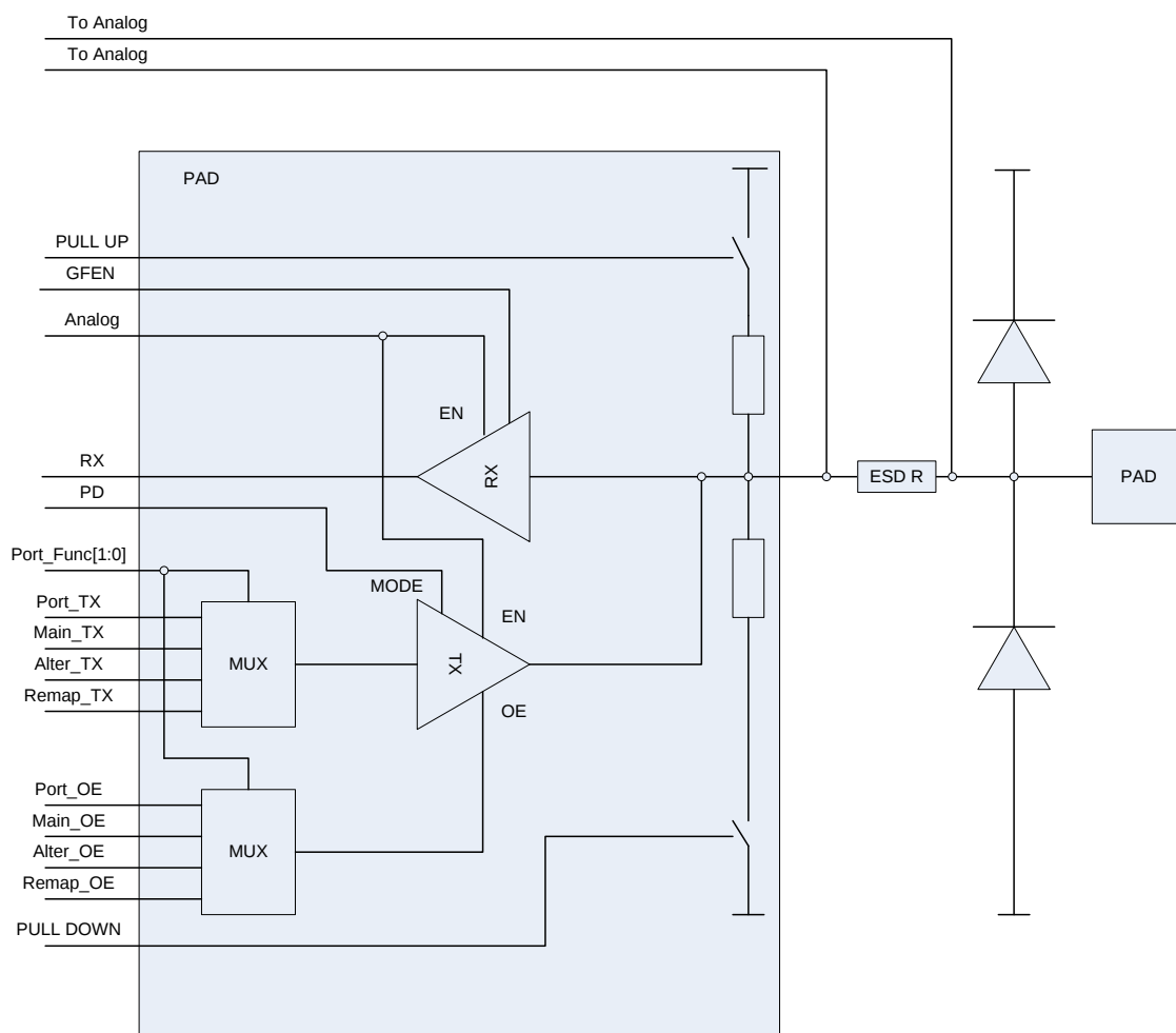
Рисунок 30 – Структурная схема
