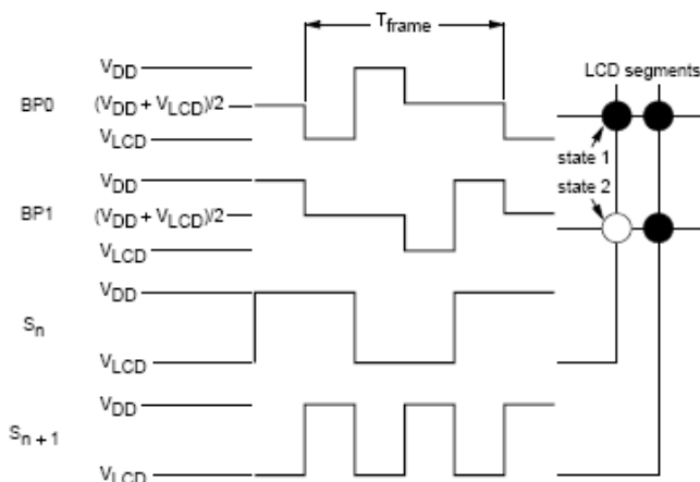
Рисунок 86 – Режим управления с мультиплексом 1:2 и 1/2 bias
