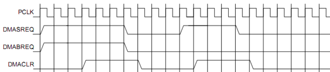
Рисунок 82 – Временные диаграммы одноэлементного и блочного запросов DMA
