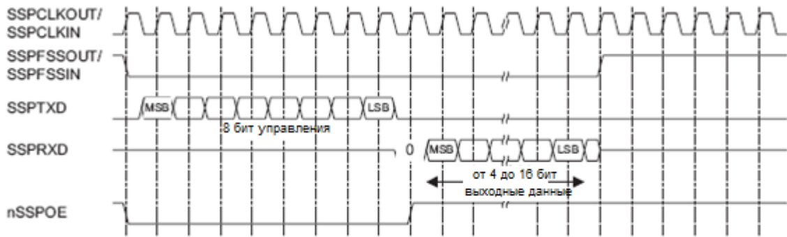
Рисунок 69 – Формат синхронного обмена протокола Microwire фирмы National Semiconductor (одиночный обмен)
