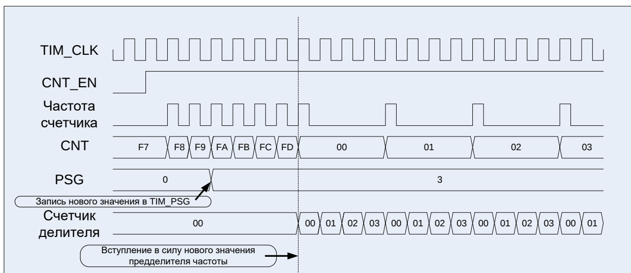
Рисунок 37 – Диаграммы работы счетчика: счет вверх (CNT_MODE = 00, EVENT_SEL = 0000, DIR = 0)
