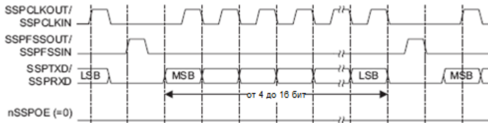
Рисунок 64 – Формат синхронного обмена протокола SPI фирмы Motorola, SPO=0, SPH=0 (непрерывный обмен)
