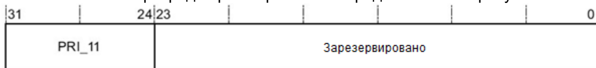
Рисунок 101 – Назначение разрядов регистра SHPR2
