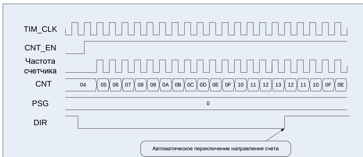
Рисунок 34 – Диаграммы работы таймера, счет вверх/вниз, сначала вверх
