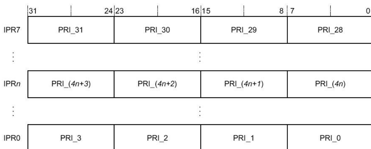
Рисунок 95 – Поля приоритетов регистров IPR0-IPR7
