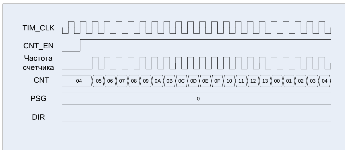
Рисунок 32 – Диаграммы работы таймера, счет вверх от 0 до 0x0013, стартовое значение 0x0004
