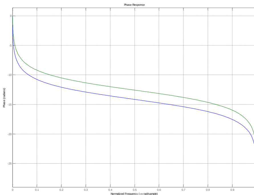
Рисунок 23 – Фильтр для сдвига сигнала на 90 градусов
