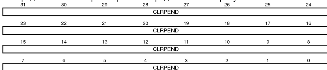
Рисунок 94 – Распределение битов регистра ICPR
