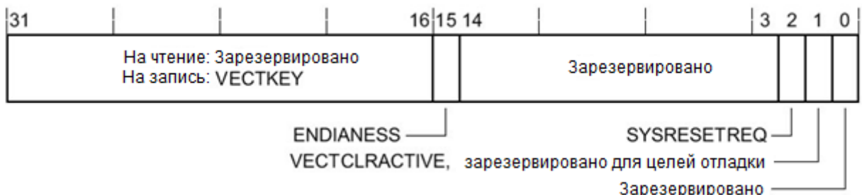
Рисунок 98 – Назначение разрядов регистра AIRCR
