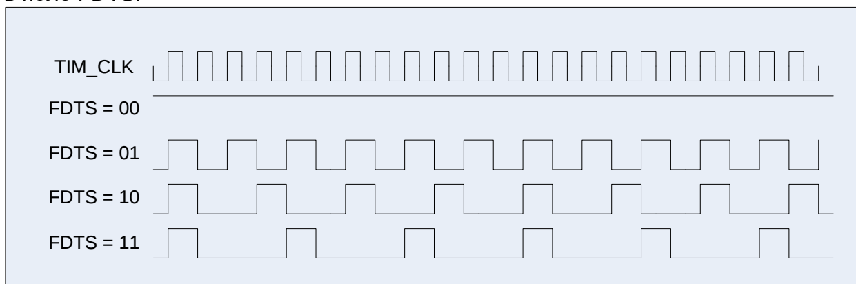
Рисунок 42 – Диаграммы возможных частот семплирования данных (FDTS)
