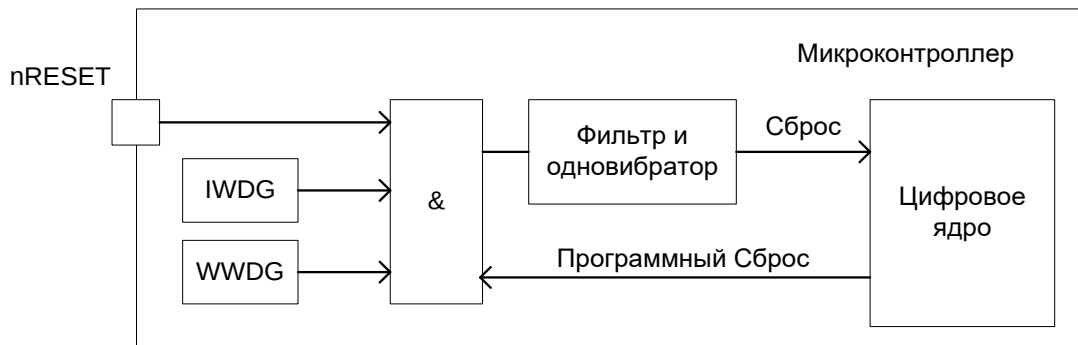
Рисунок 4 – Схема формирования сигнала сброса
