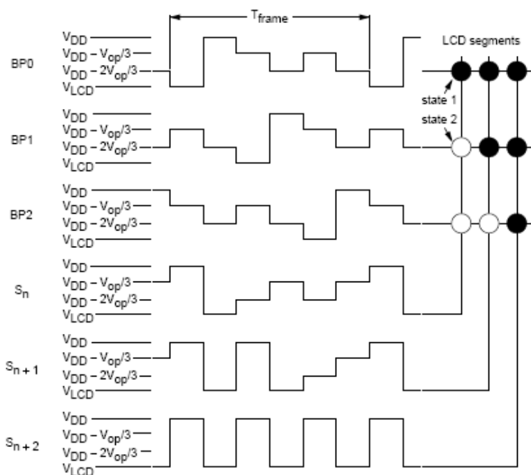
Рисунок 88 – Режим управления с мультиплексом 1:3
