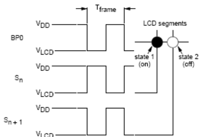
Рисунок 85 – Статический режим управления
