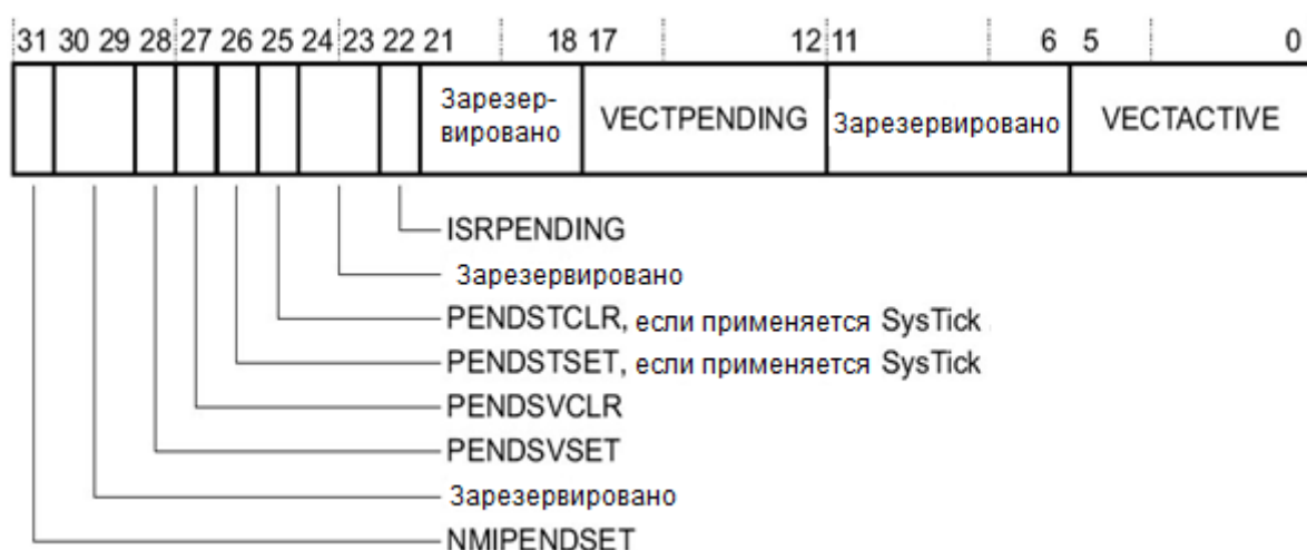
Рисунок 97 – Назначение разрядов регистра ICSR
