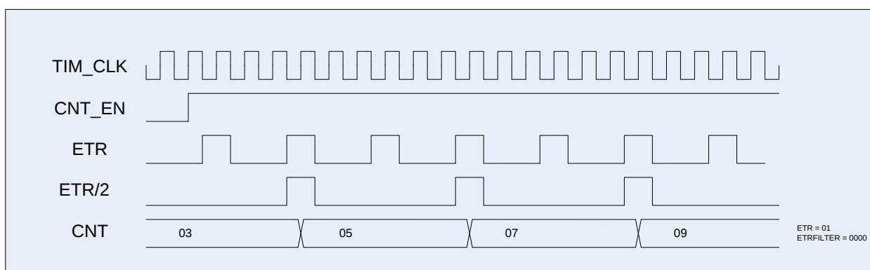
Рисунок 47 – Диаграмма тактирования сигналом со входа ETR
