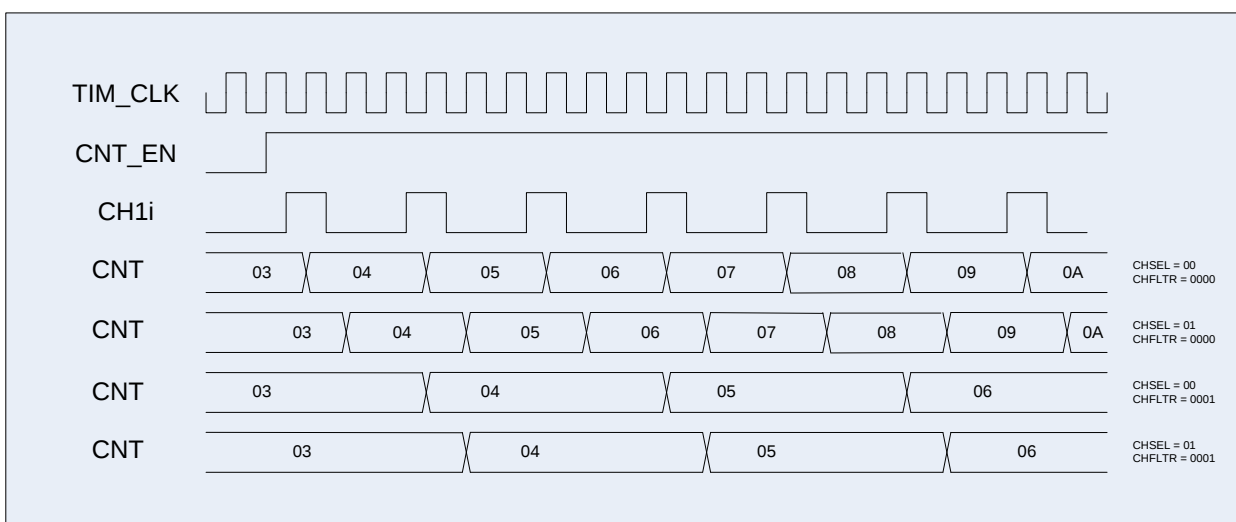
Рисунок 44 – Диаграмма внешнего тактирования с разными вариантами фильтра
