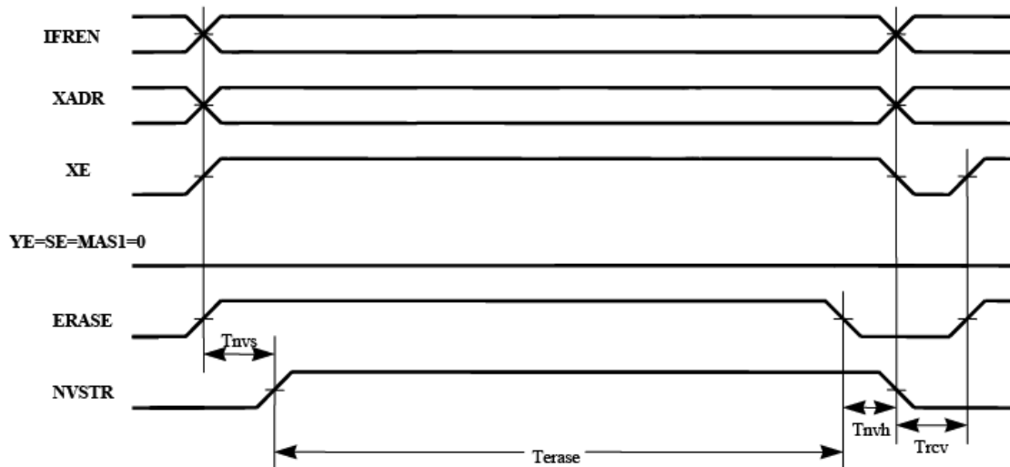
Рисунок 9 – Временная диаграмма стирания страницы
