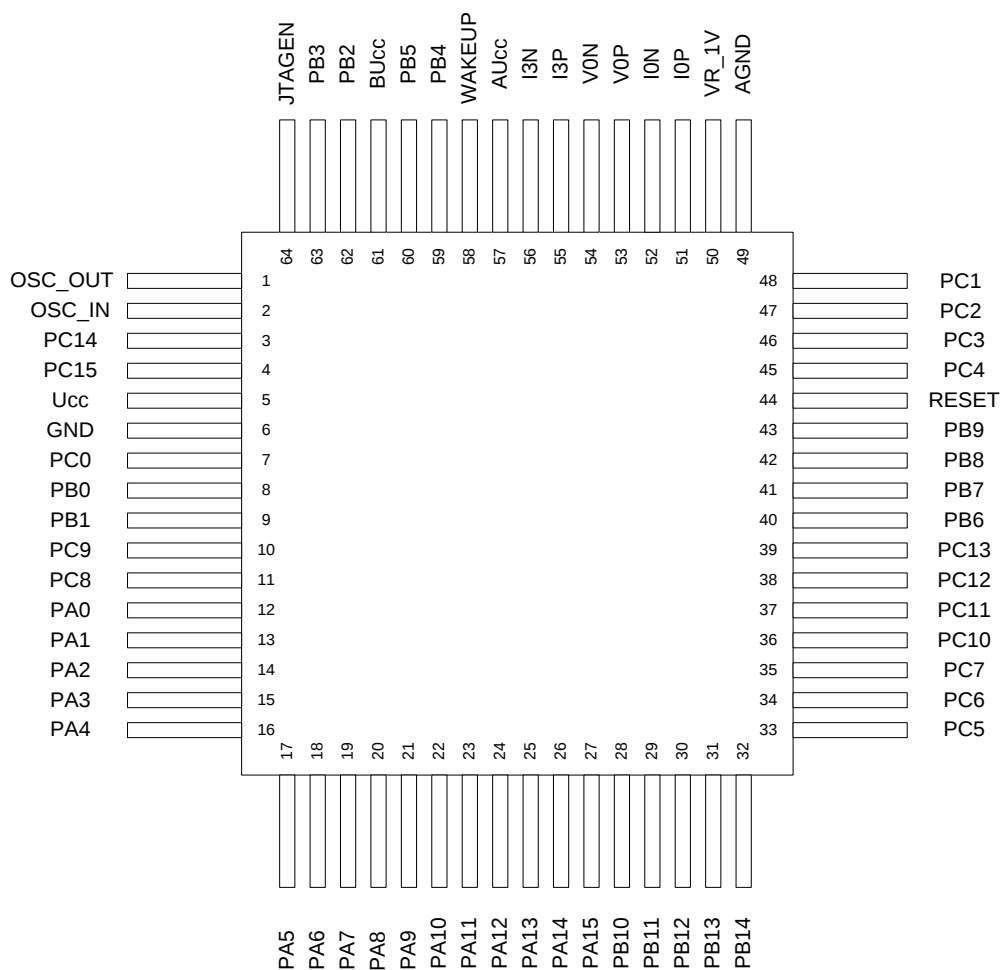
Рисунок 1 – 64-выводной пластиковый корпус LQFP64
