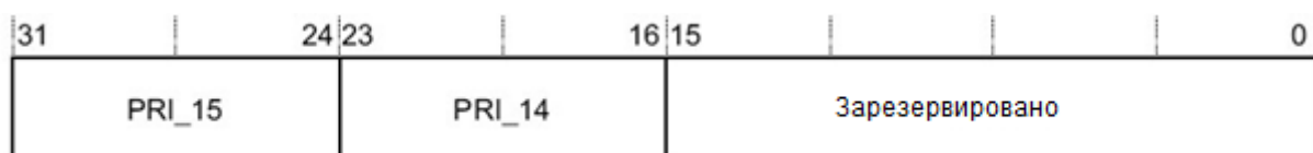
Рисунок 102 – Назначение разрядов регистра SHPR3
