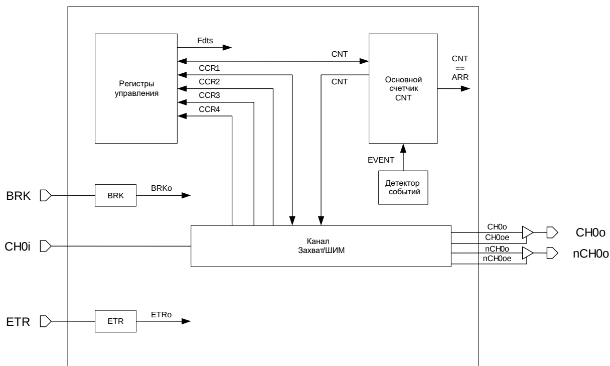
Рисунок 31 – Структурная схема таймера
