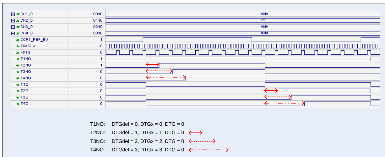
Рисунок 54 – Диаграмма работы схемы DTG
