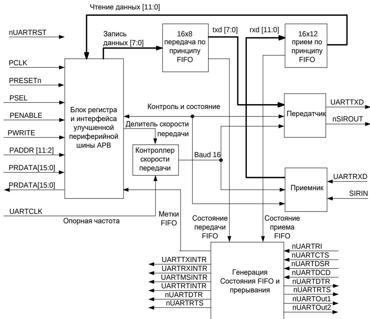
Рисунок 76 – Блок-схема универсального асинхронного приёмопередатчика (УАПП)
