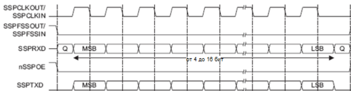
Рисунок 65 – Формат синхронного обмена протокола SPI фирмы Motorola, SPO=0, SPH=1
