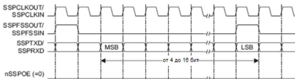
Рисунок 62 – Формат синхронного обмена протокола SSI фирмы Texas Instruments (непрерывный обмен)
