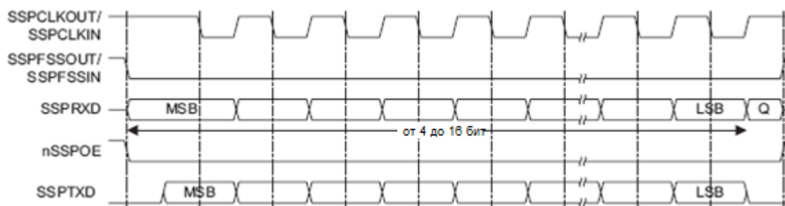
Рисунок 66 – Формат синхронного обмена протокола SPI фирмы Motorola, SPO=1, SPH=0 (одиночный обмен)
