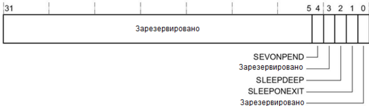
Рисунок 99 – Назначение разрядов регистра SCR
