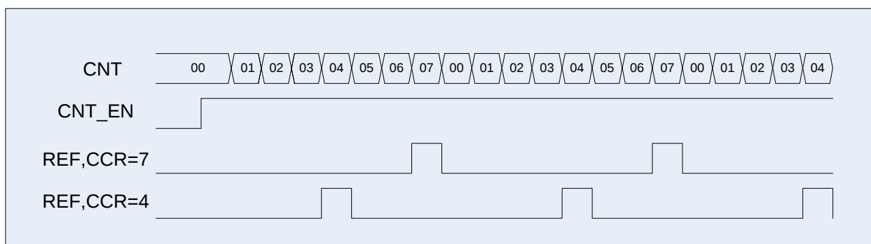
Рисунок 51 – Диаграмма работы схемы в режиме ШИМ, CCR1_EN=0
