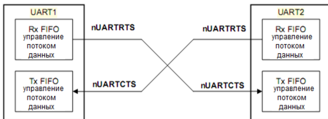
Рисунок 81 – Взаимодействие двух устройств последовательной связи с аппаратным управлением потоком данных
