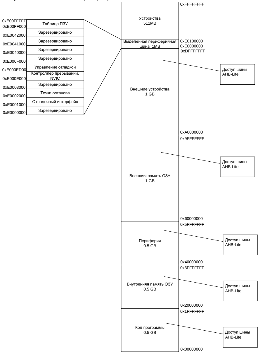
Рисунок 6 – Адресное пространство микроконтроллера
