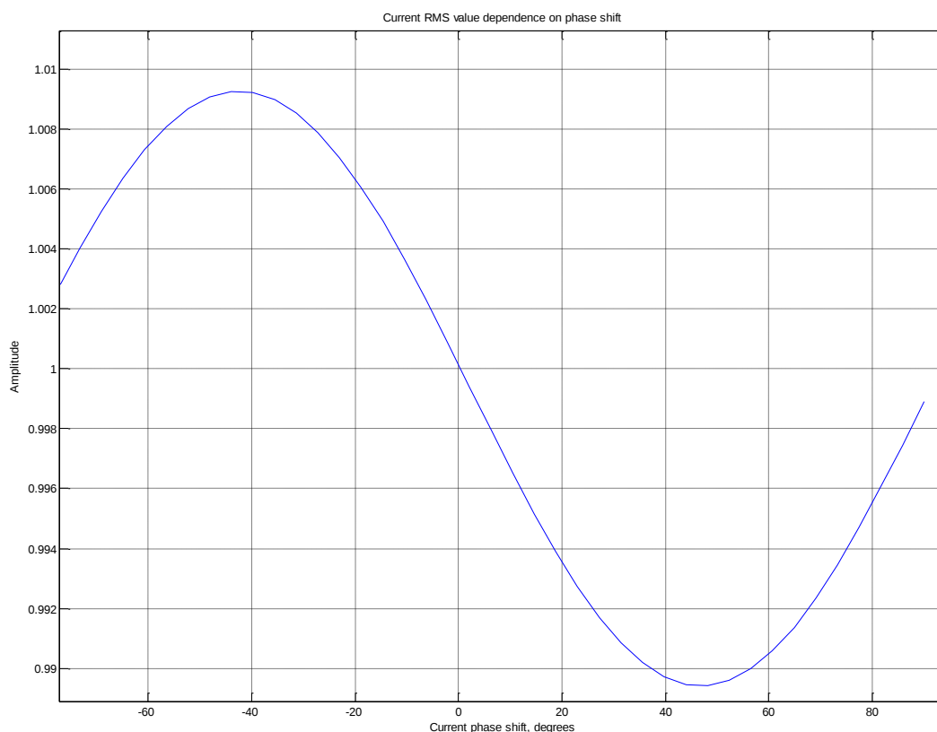
Рисунок 17 – Зависимость действующего значения тока от фазового сдвига
