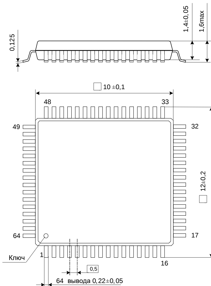
Рисунок 103 – Корпус LQFP64
