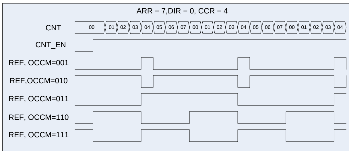
Рисунок 52 – Диаграмма работы схемы в режиме ШИМ, CCR1_EN=0
