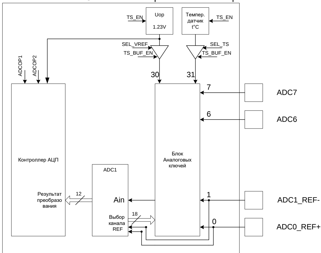
Рисунок 59 – Структурная схема контроллера АЦП
