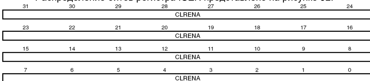
Рисунок 92 – Распределение битов регистра ICER
