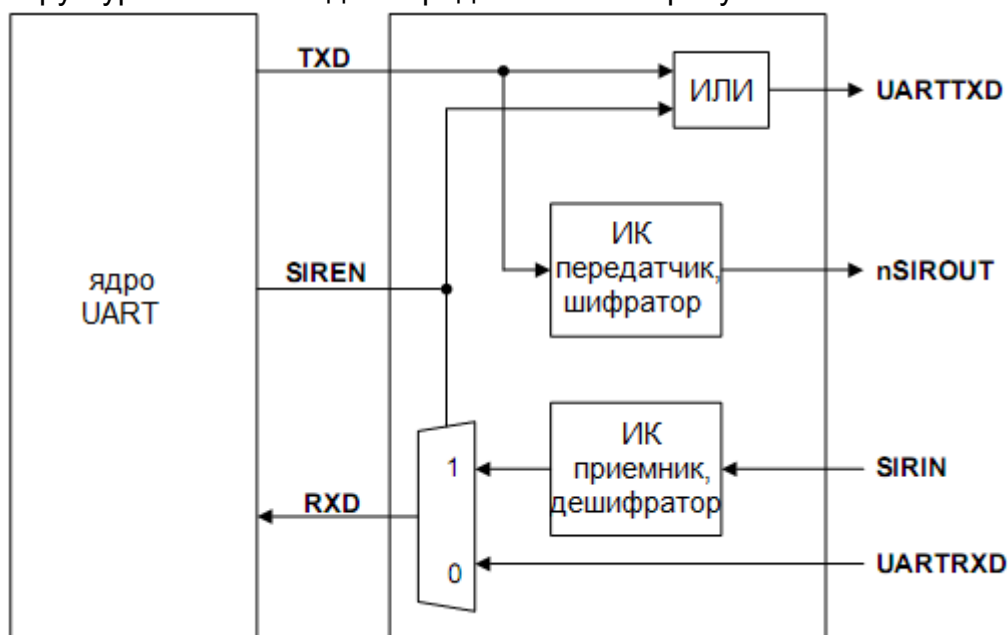
Рисунок 77 – Структурная схема кодака
