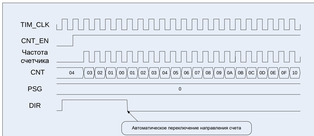
Рисунок 35 – Диаграммы работы таймера, счет вверх/вниз, сначала вниз
