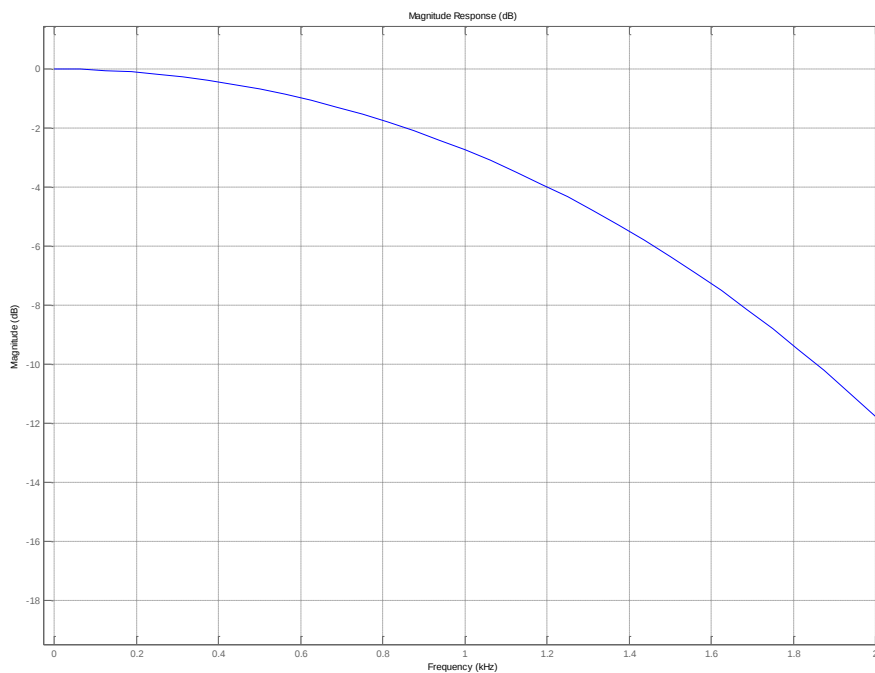
Рисунок 21 – Характеристика децимирующего фильтра в полосе 2 кГц
