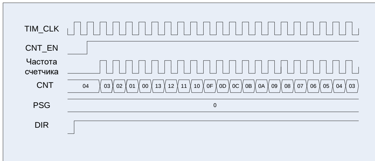
Рисунок 33 – Диаграммы работы таймера, счет вниз от 0x0013 до 0, стартовое значение 0x0004
