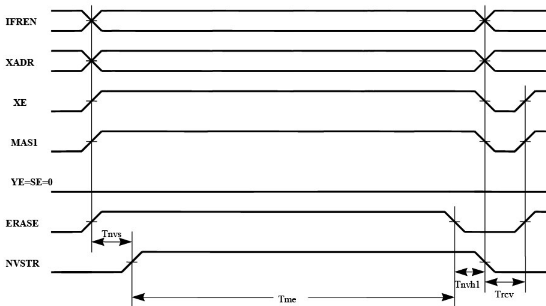
Рисунок 8 – Временная диаграмма стирания памяти
