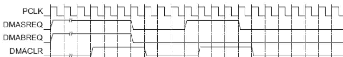
Рисунок 75 – Временные диаграммы обмена в режиме ПДП
