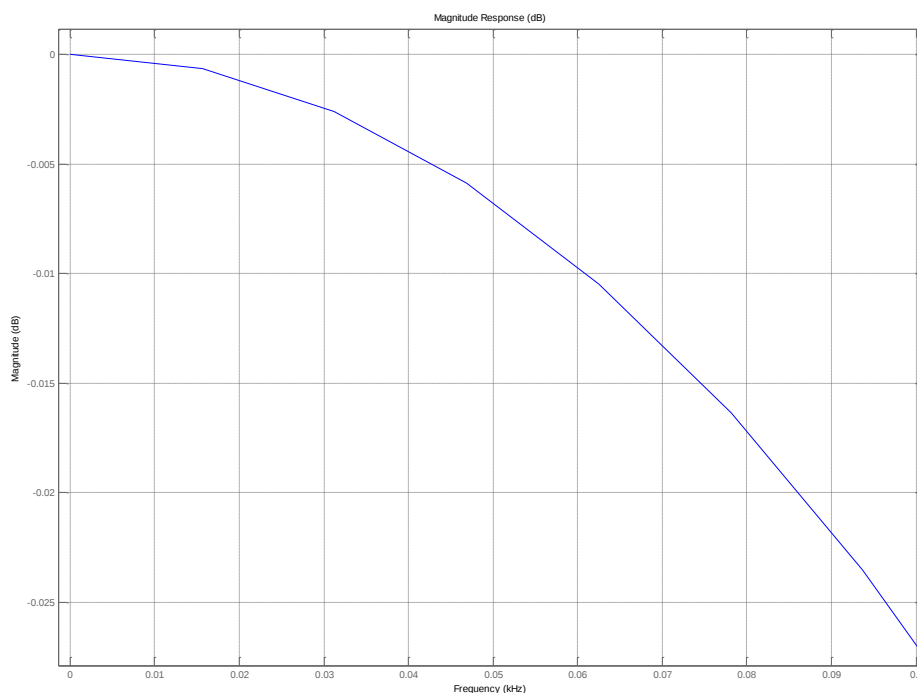
Рисунок 22 – Характеристика децимирующего фильтра в полосе 100 Гц
