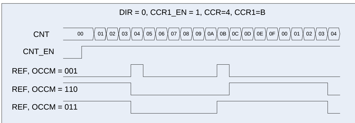
Рисунок 55 – Диаграмма работы схемы в режиме ШИМ, CCR1_EN = 1
