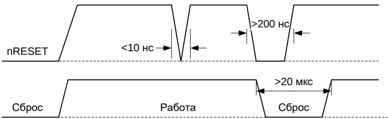
Рисунок 5 – Временная диаграмма формирования сигнала сброса
