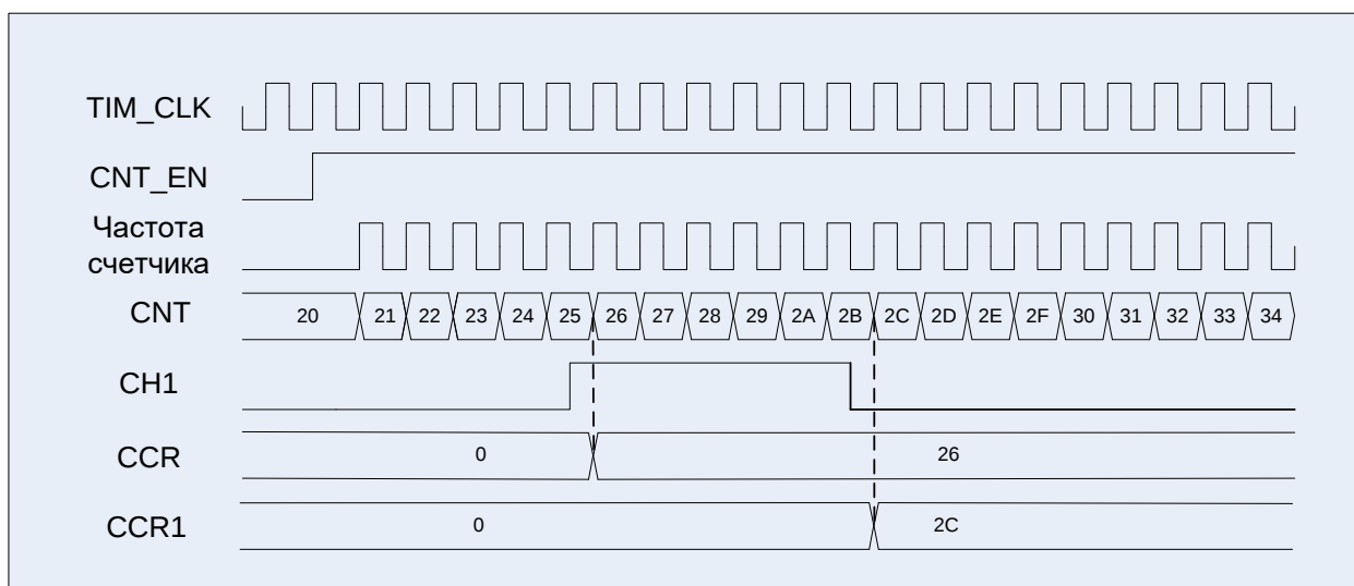
Рисунок 49 – Диаграмма захвата события со входа первого канала
