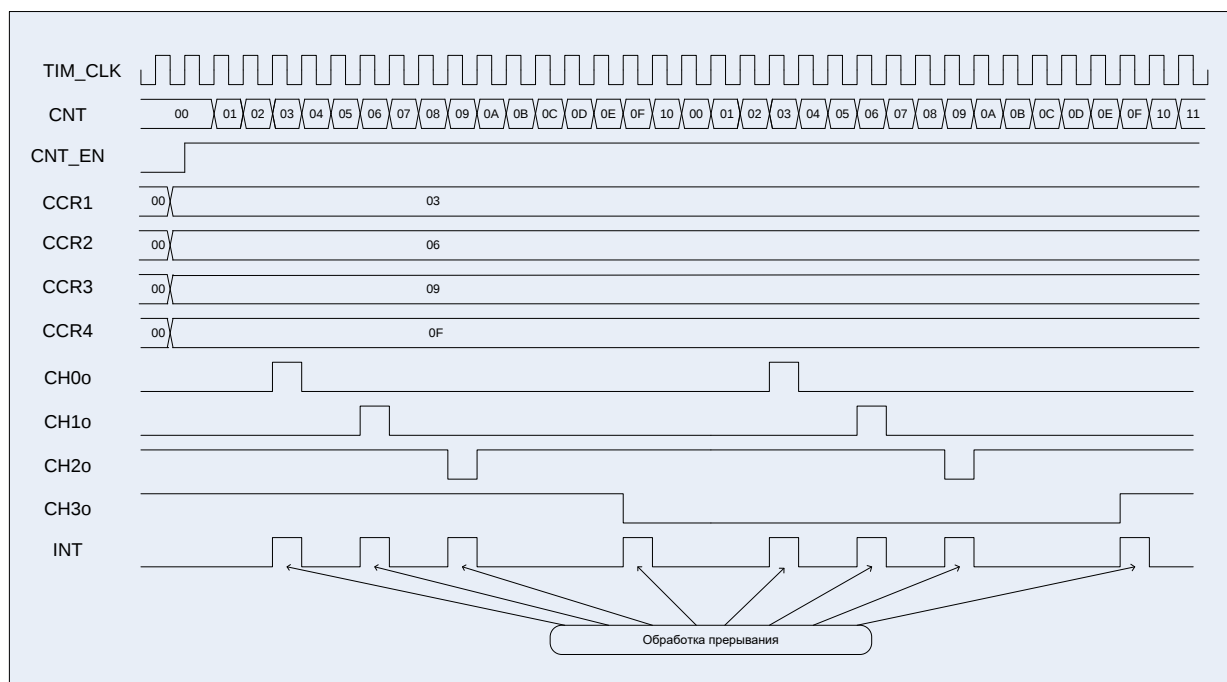
Рисунок 58 – Диаграммы примера работы в режиме ШИМ
