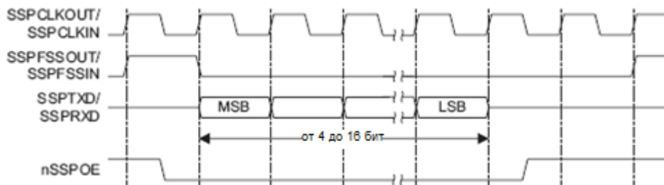
Рисунок 61 – Формат синхронного обмена протокола SSI фирмы Texas Instruments (единичный обмен)
