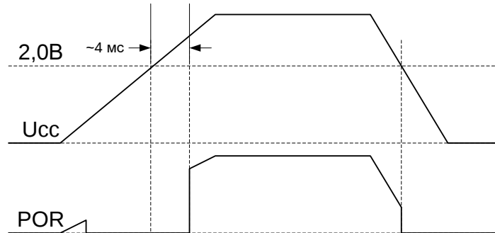
Рисунок 1 – Схема включения основного питания U_{cc}
