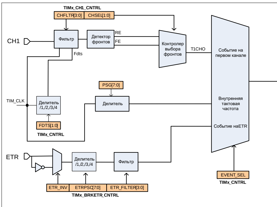
Рисунок 36 – Структурная схема формирования события для счета
