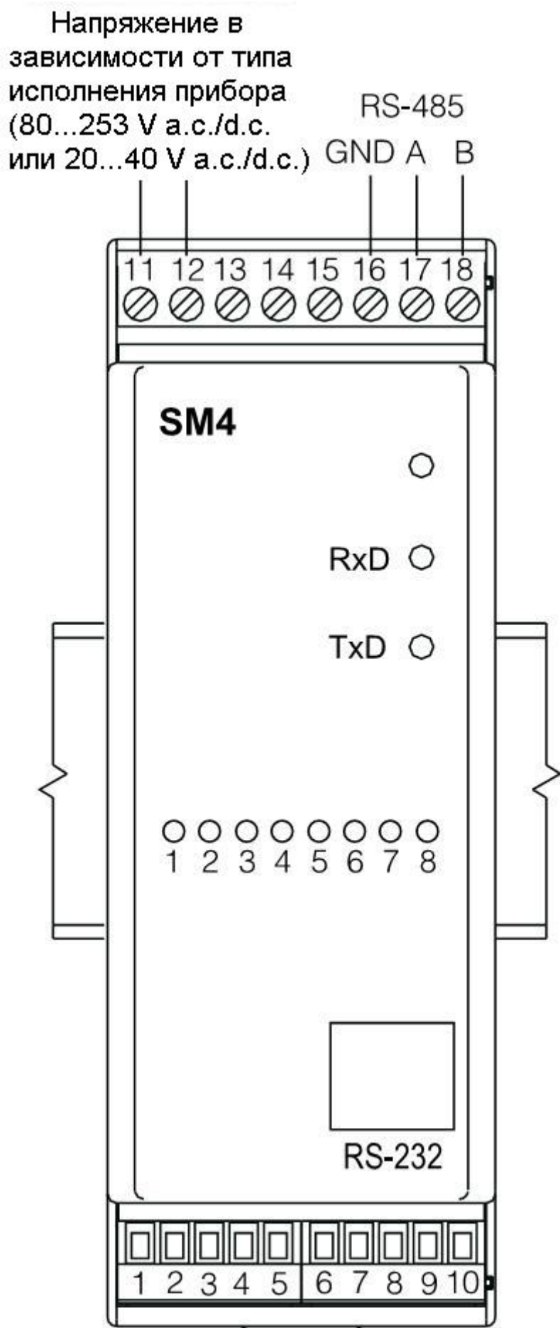
Рис.3. Схема электрических соединений для модуля SM4
