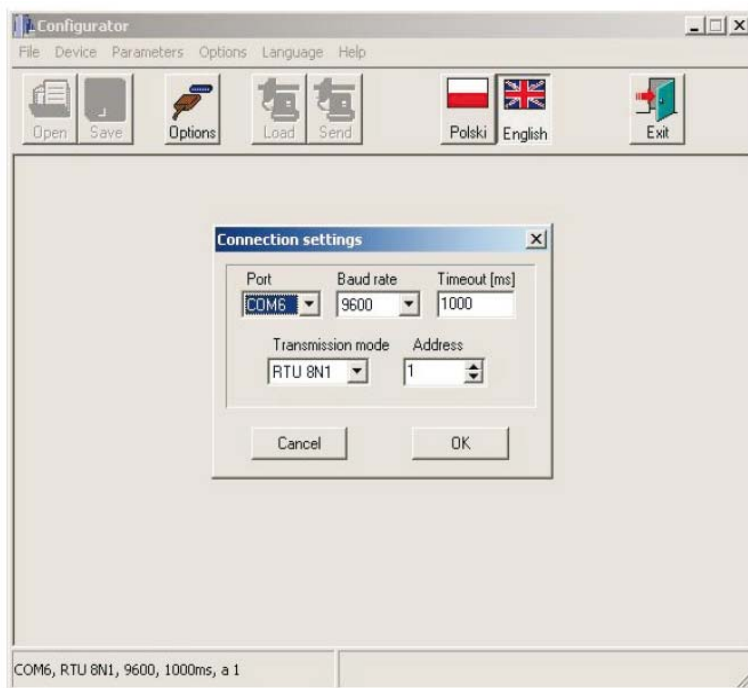
Рис.3. Конфигурирование соединения с преобразователем P20
