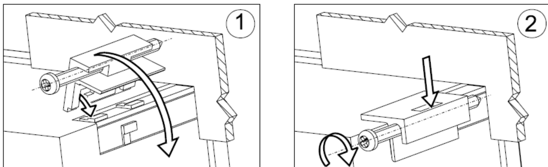
Рис. 2. Установка прибора на щит
