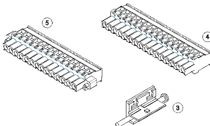
Fig.1, Meter set
