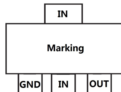
SOT-89
