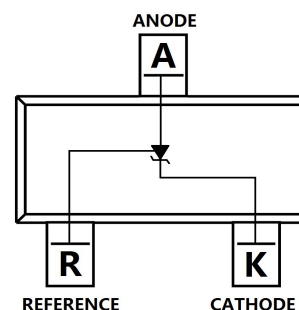
SOT-23
