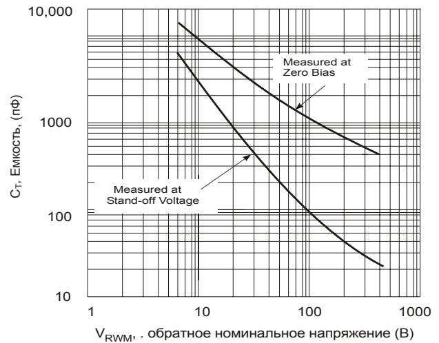
Рис.1 - Типичная общая емкость
