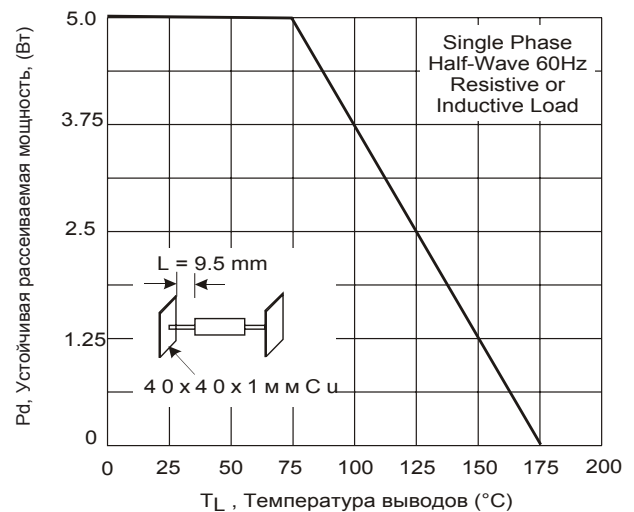
Рис.5 - Кривая уменьшения мощности
