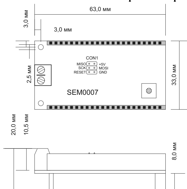
Габаритный чертеж
