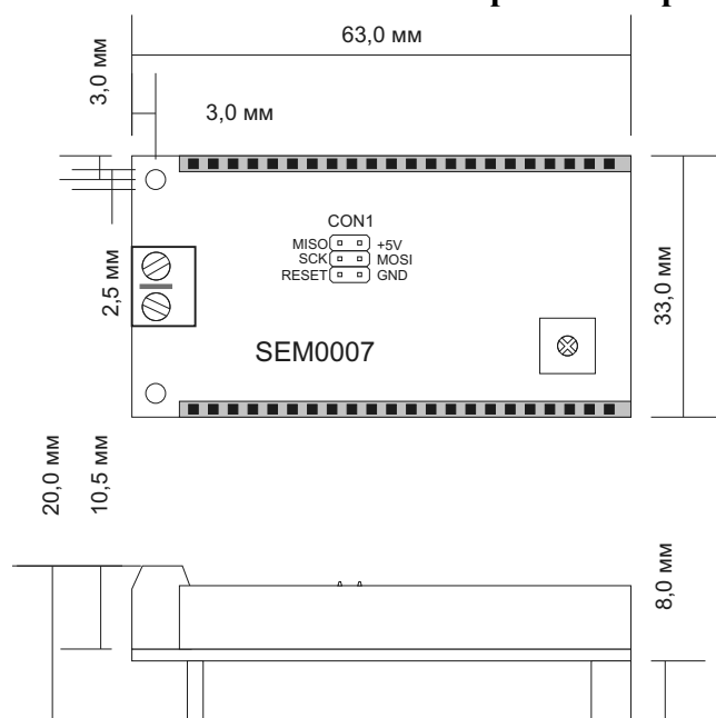
Габаритный чертеж
