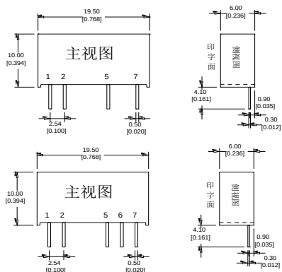
封装尺寸图
