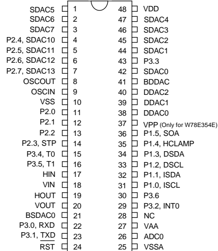
W78C/E354E (DIP48)
