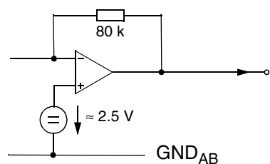
Fig. 6-26: Output pins AOUT1, AOUT2
