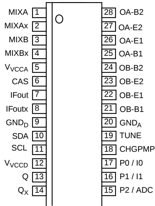
P-TSSOP 28-1
