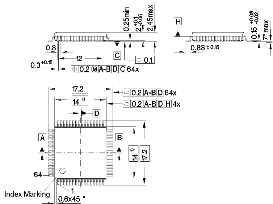
P-MQFP 64-1
