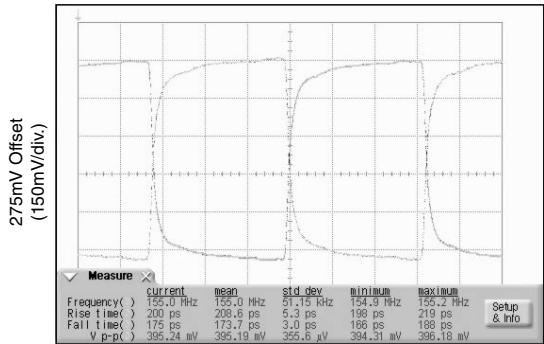
155MHz Output
