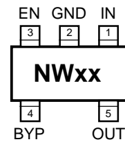
MIC5255-x.xBD5 (TSOT-23-5)
