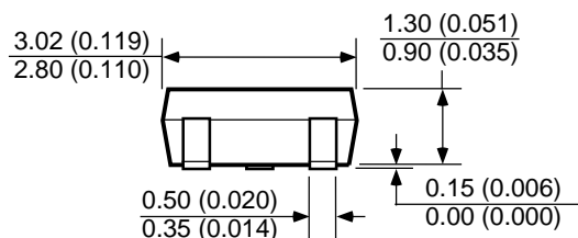
SOT-23-5 (M5)
