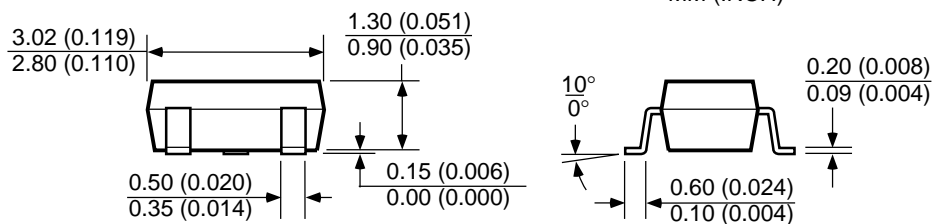
SOT-23-5 (M)
