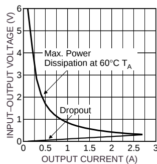
Si3445DV SOA
