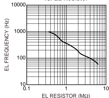
EL Frequency vs. EL Resistor
