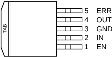
TO-263-5 (U)
