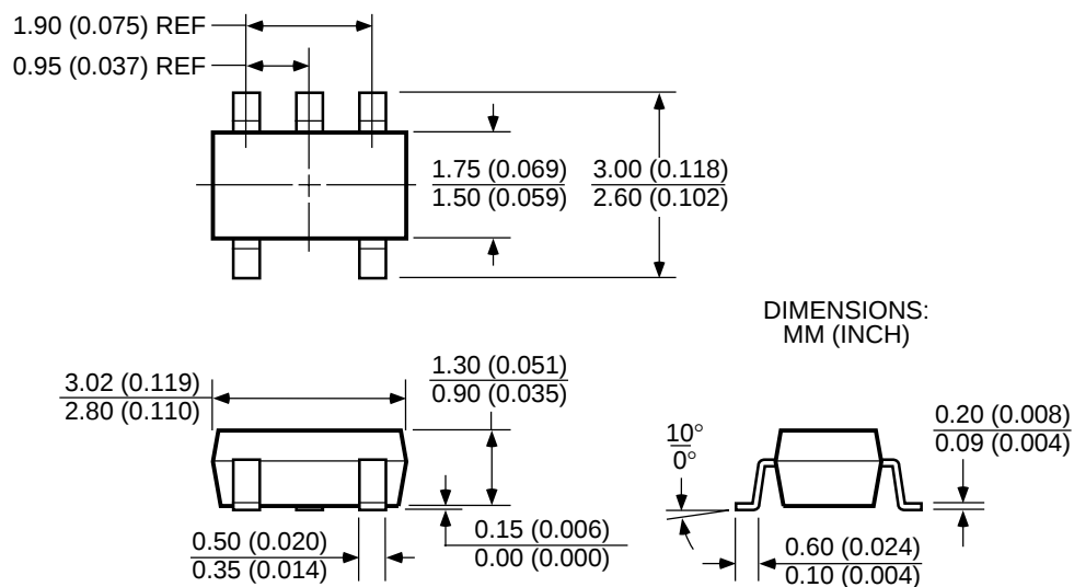
SOT-23-5 (M)
