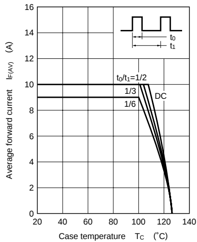
I_{F(AV)} - T_C
