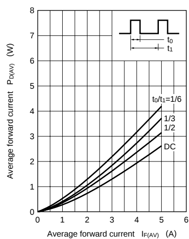
P_{D(AV)} - I_{F(AV)}
