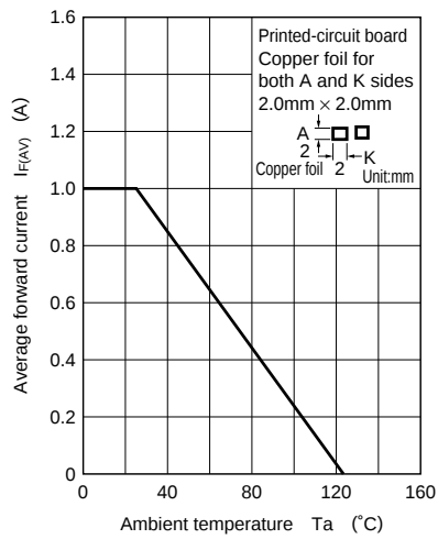
I_{F(AV)} - T_a
