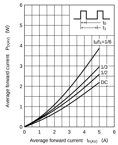
P_{D(AV)} - I_{F(AV)}
