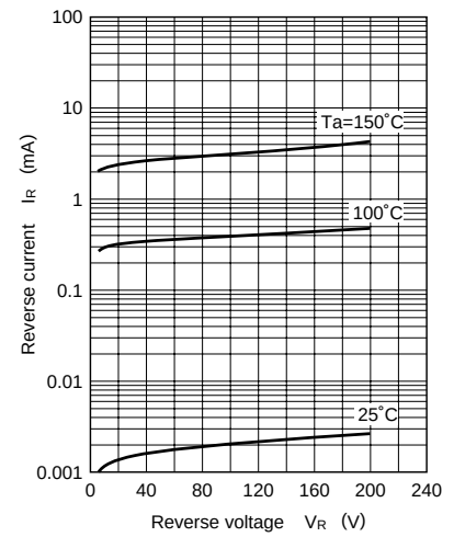
I_R - V_R
