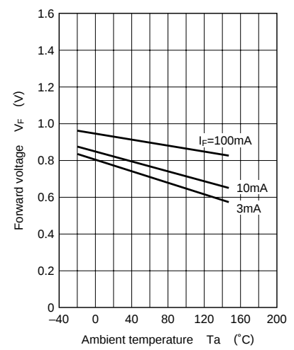
V_F - T_a
